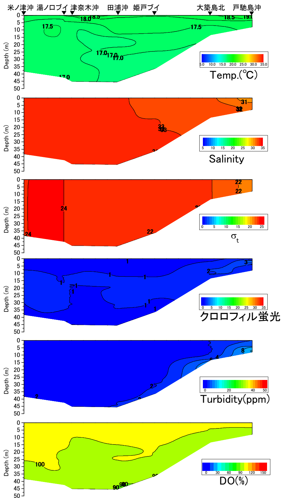
戸馳島沖から米ノ津沖の水温(°C)、塩分、密度( \sigma_t )、クロロフィル蛍光強度、濁度、溶存酸素飽和度(DO%)の鉛直面図(熊本県水産研究センターの調査による)(2017年5月1日)
