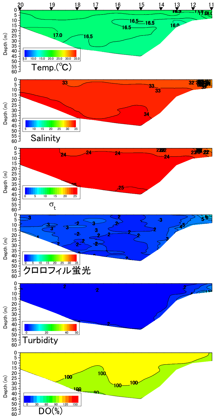
八代海中央ラインの水温(°C)、塩分、密度( \sigma_t )、クロロフィル蛍光強度、濁度、溶存酸素飽和度(DO%)の鉛直面図(国土交通省の調査による) (2017年4月26日)
