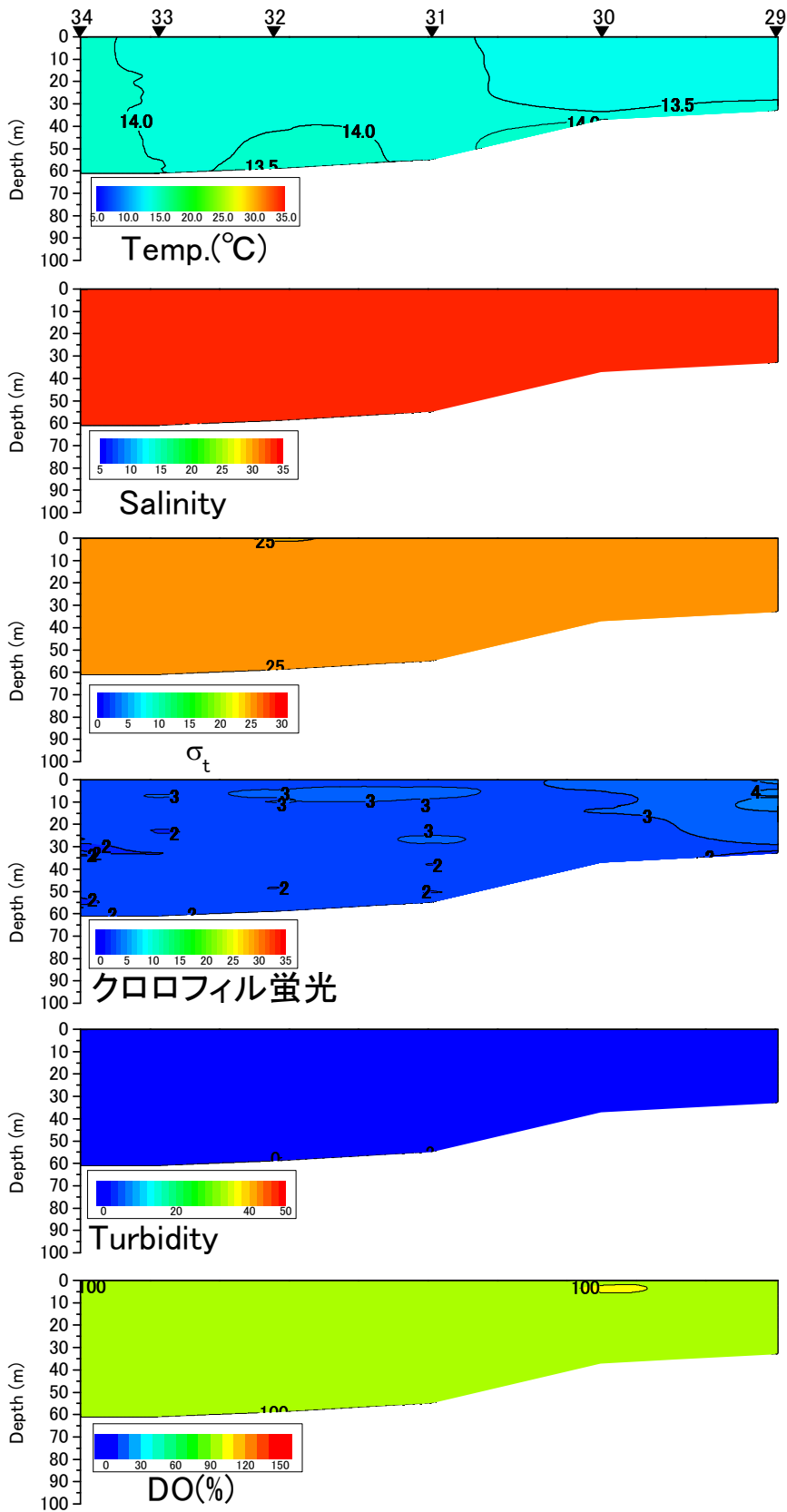
八代海西ラインの水温(°C)、塩分、密度( \sigma_t )、クロロフィル蛍光強度、濁度、溶存酸素飽和度(DO%)の鉛直面図(国土交通省の調査による) (2017年3月8日)
