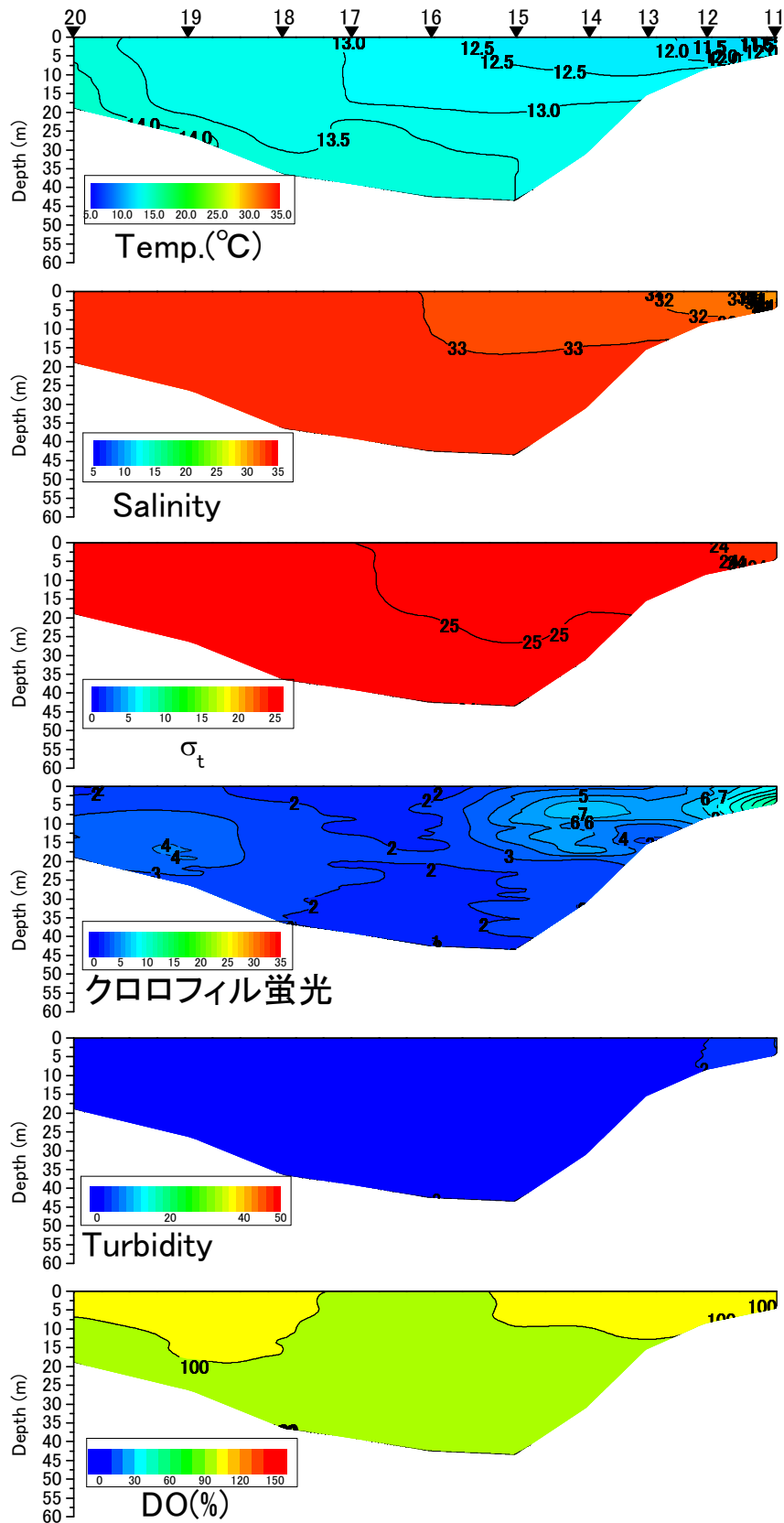
八代海中央ラインの水温(°C)、塩分、密度( \sigma_t )、クロロフィル蛍光強度、濁度、溶存酸素飽和度(DO%)の鉛直面図(国土交通省の調査による) (2017年3月7日)
