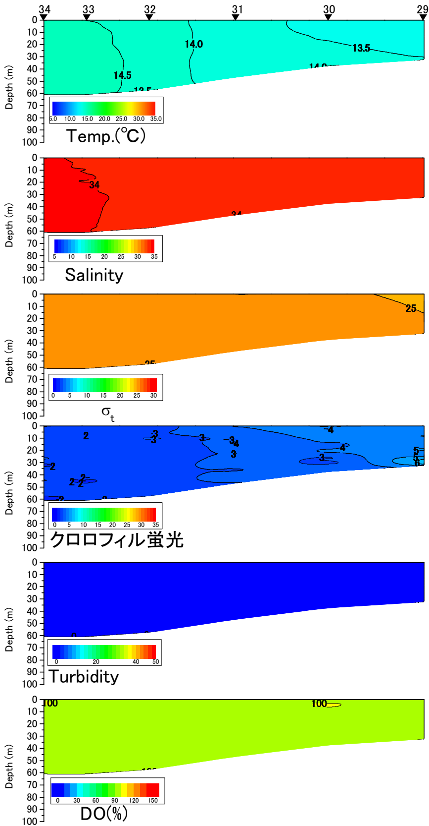
八代海西ラインの水温(°C)、塩分、密度( \sigma_t )、クロロフィル蛍光強度、濁度、溶存酸素飽和度(DO%)の鉛直面図(国土交通省の調査による) (2017年3月1日)
