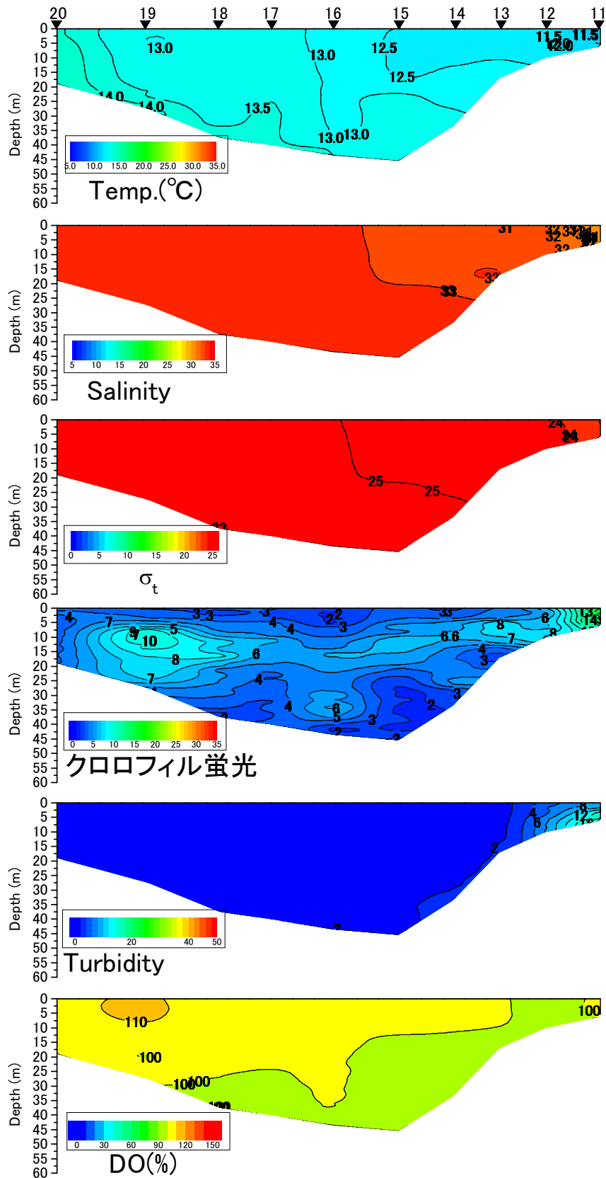
八代海中央ラインの水温(°C)、塩分、密度( \sigma_t )、クロロフィル蛍光強度、濁度、溶存酸素飽和度(DO%)の鉛直面図(国土交通省の調査による) (2017年2月28日)
