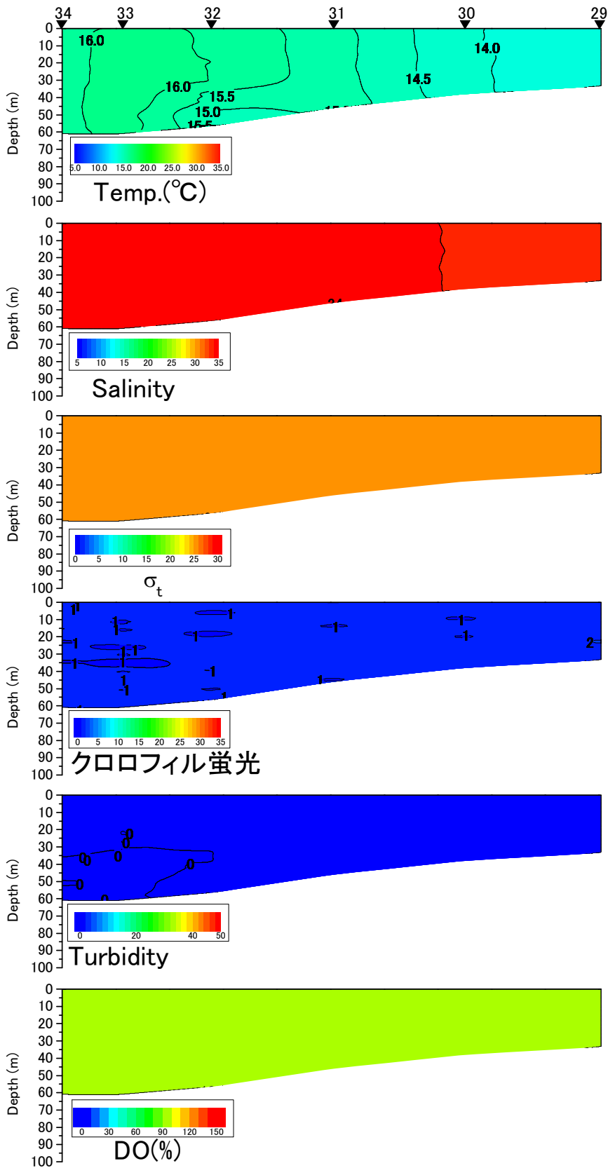
八代海西ラインの水温(°C)、塩分、密度( \sigma_t )、クロロフィル蛍光強度、濁度、溶存酸素飽和度(DO%)の鉛直面図(国土交通省の調査による) (2017年2月10日)
