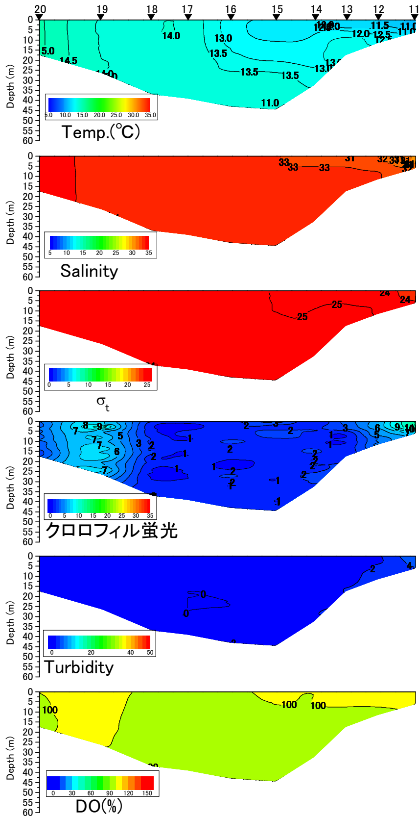
八代海中央ラインの水温(°C)、塩分、密度( \sigma_t )、クロロフィル蛍光強度、濁度、溶存酸素飽和度(DO%)の鉛直面図(国土交通省の調査による) (2017年2月9日)
