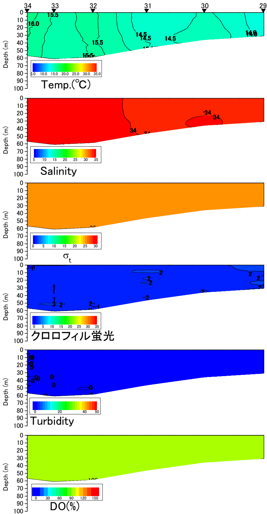
八代海西ラインの水温(°C)、塩分、密度( \sigma_t )、クロロフィル蛍光強度、濁度、溶存酸素飽和度(DO%)の鉛直面図(国土交通省の調査による) (2017年2月3日)
