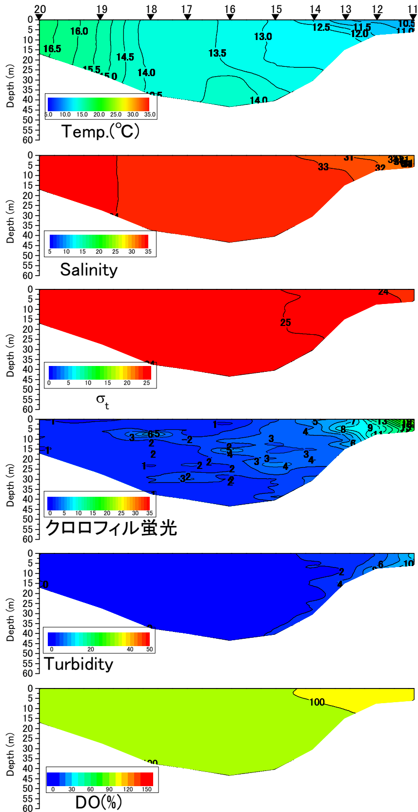
八代海中央ラインの水温(°C)、塩分、密度( \sigma_t )、クロロフィル蛍光強度、濁度、溶存酸素飽和度(DO%)の鉛直面図(国土交通省の調査による) (2017年2月2日)
