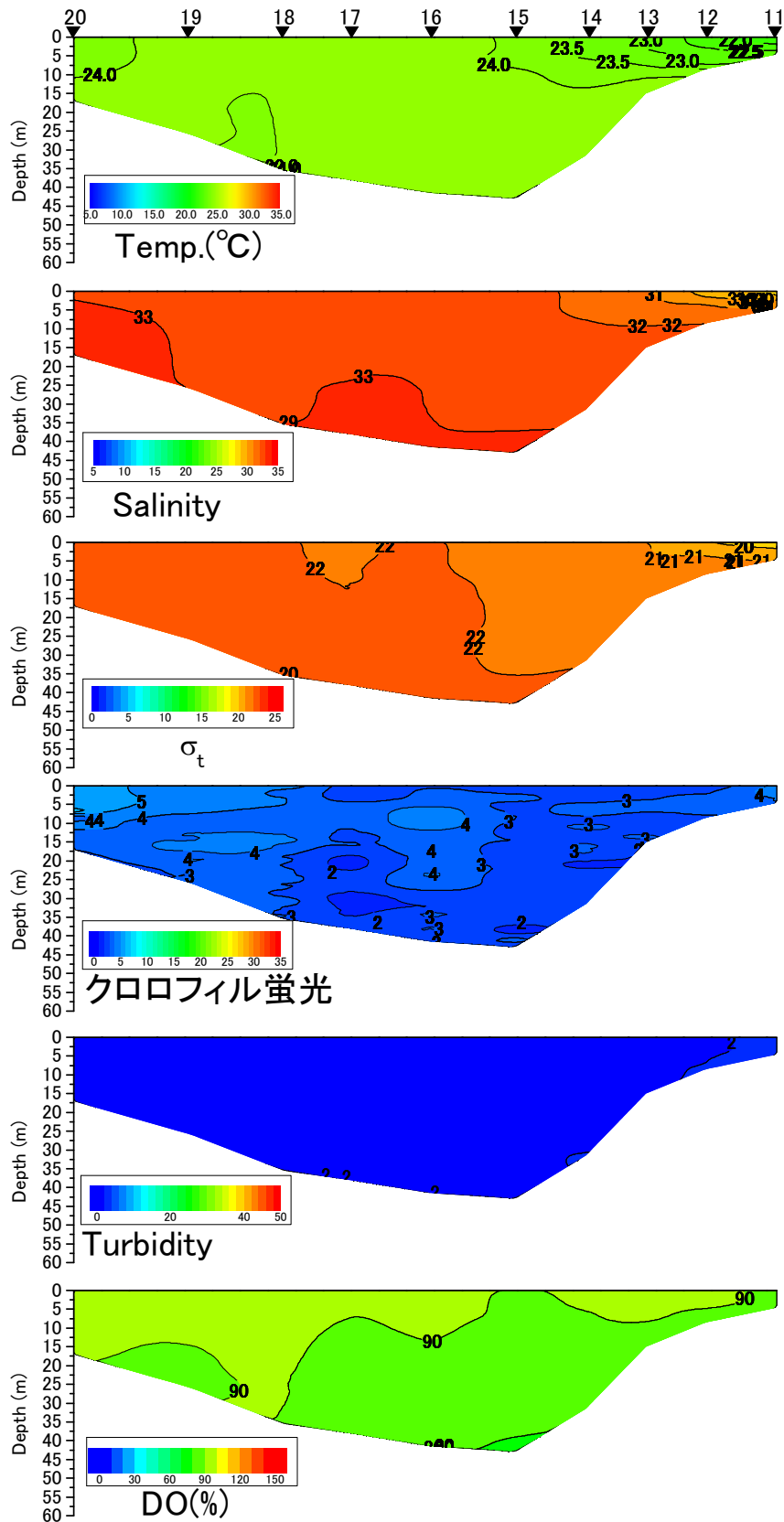
八代海中央ラインの水温(°C)、塩分、密度( \sigma_t )、クロロフィル蛍光強度、濁度、溶存酸素飽和度(DO%)の鉛直面図(国土交通省の調査による) (2016年10月25日)
