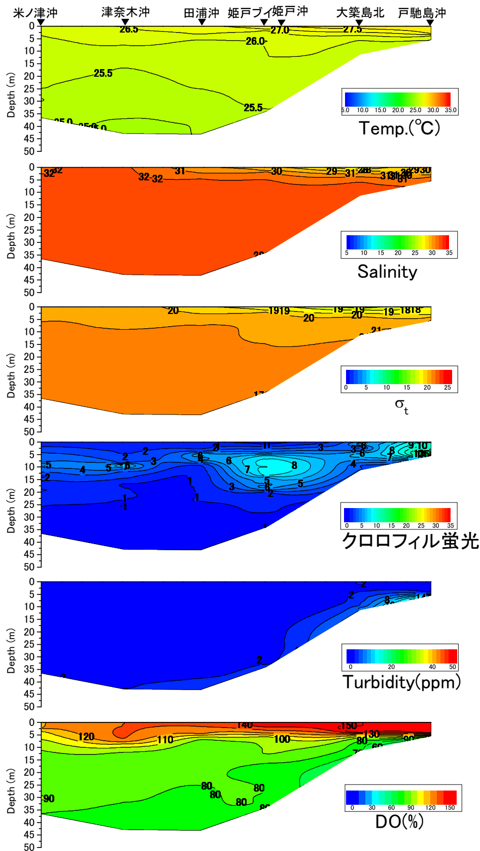
戸馳島沖から米ノ津沖の水温(°C)、塩分、密度( \sigma_t )、クロロフィル蛍光強度、濁度、溶存酸素飽和度(DO%)の鉛直面図(熊本県水産研究センターの調査による)(2016年9月27日)
