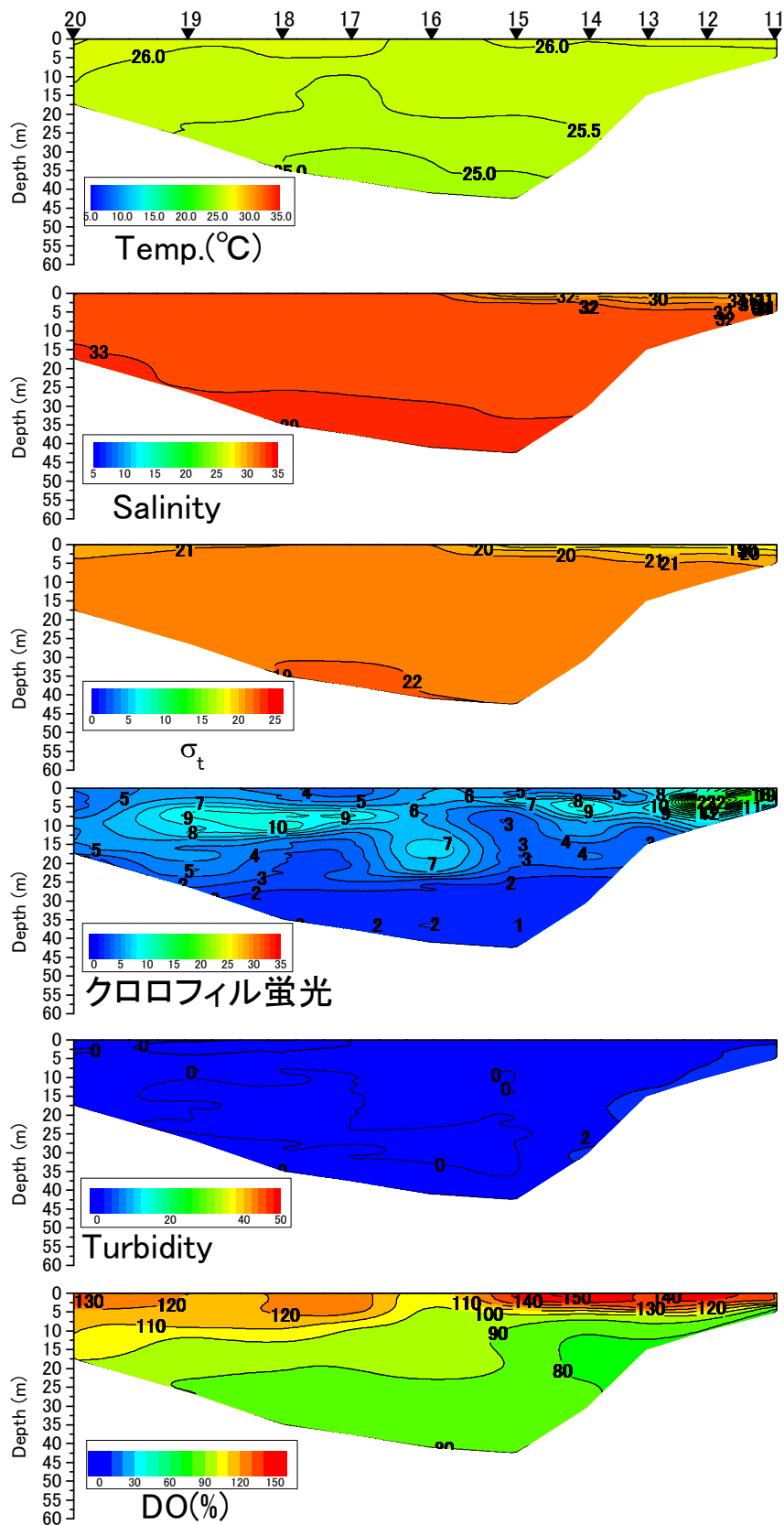
八代海中央ラインの水温(°C)、塩分、密度( \sigma_t )、クロロフィル蛍光強度、濁度、溶存酸素飽和度(DO%)の鉛直面図(国土交通省の調査による) (2016年9月26日)
