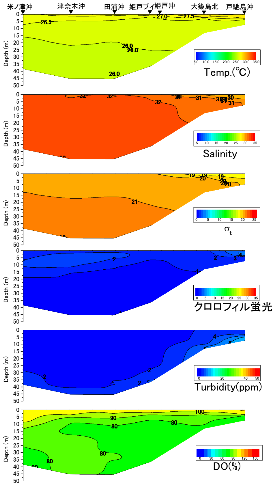
戸馳島沖から米ノ津沖の水温(°C)、塩分、密度( \sigma_t )、クロロフィル蛍光強度、濁度、溶存酸素飽和度(DO%)の鉛直面図(熊本県水産研究センターの調査による)(2016年9月6日)
