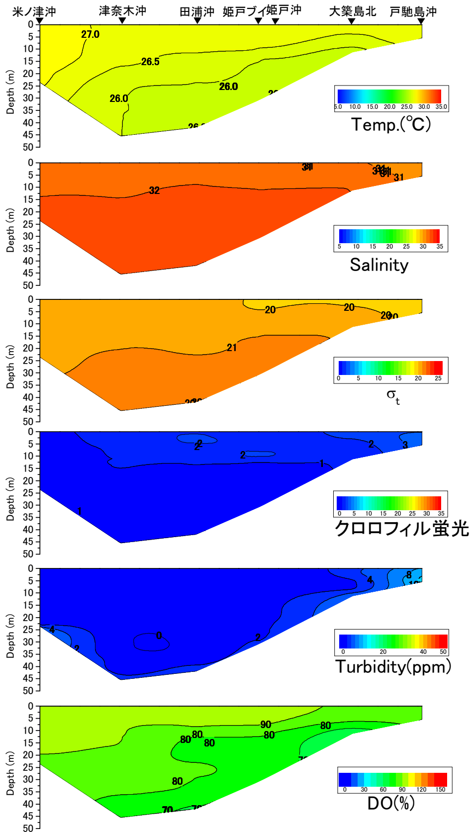
戸馳島沖から米ノ津沖の水温(°C)、塩分、密度( \sigma_t )、クロロフィル蛍光強度、濁度、溶存酸素飽和度(DO%)の鉛直面図(鹿児島県水産技術開発センターの調査による)(2016年8月29日)
