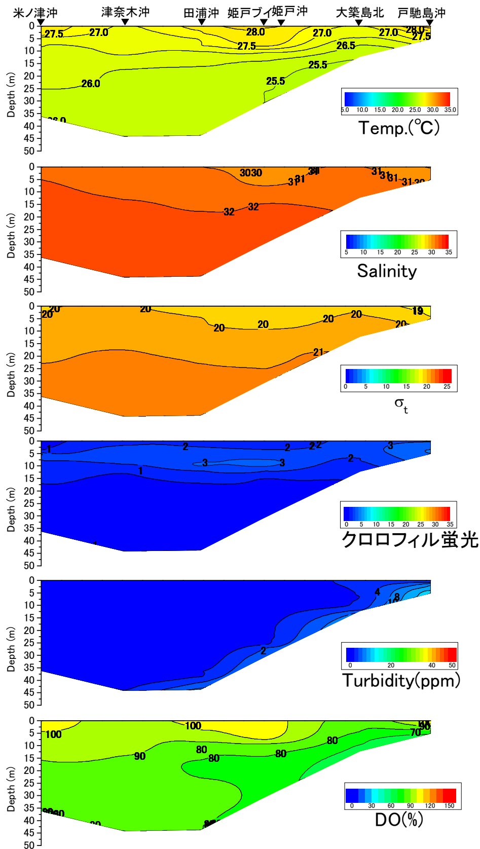
戸馳島沖から米ノ津沖の水温(°C)、塩分、密度( \sigma_t )、クロロフィル蛍光強度、濁度、溶存酸素飽和度(DO%)の鉛直面図(鹿児島県水産技術開発センターの調査による)(2016年8月24日)
