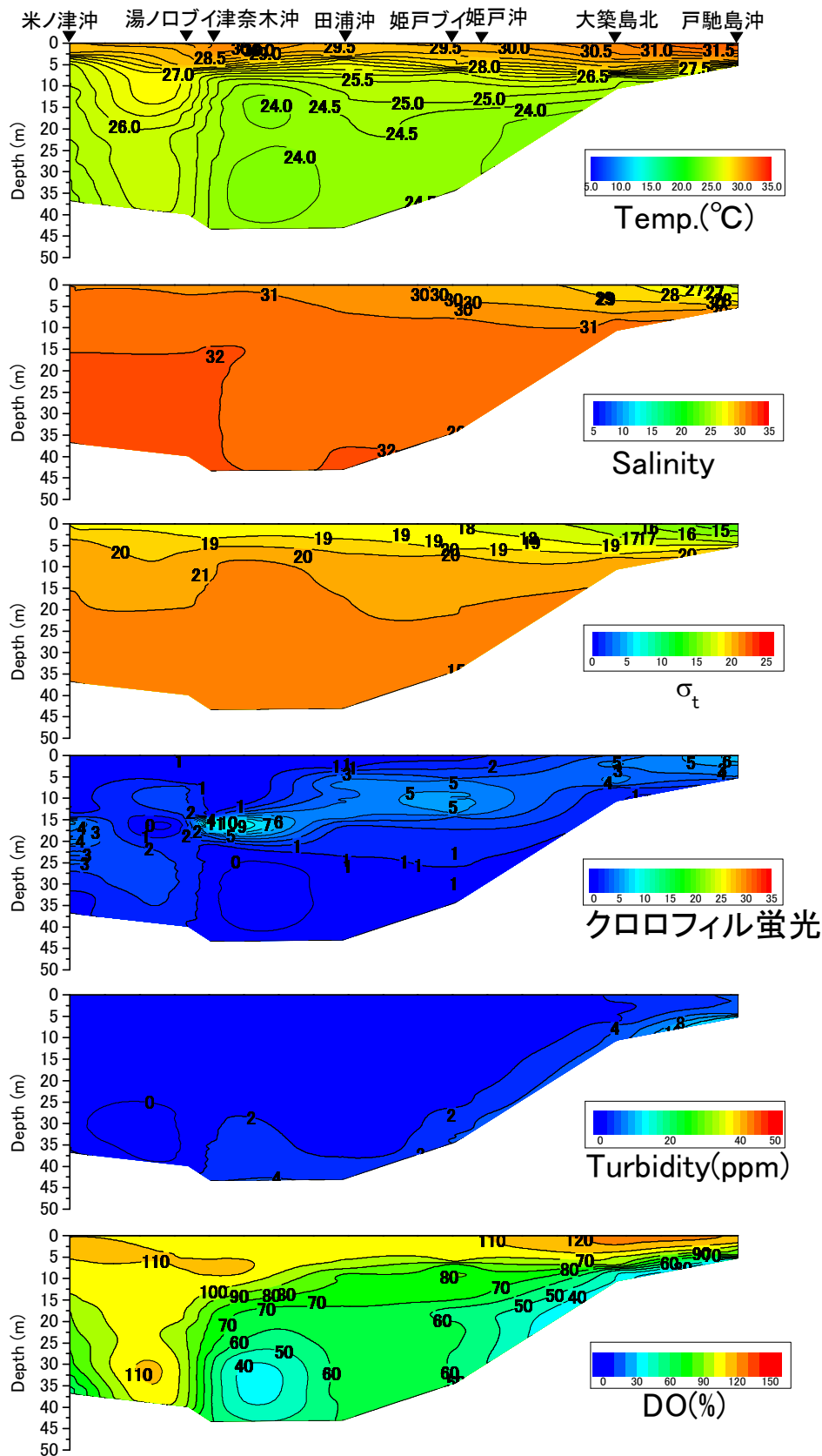
戸馳島沖から米ノ津沖の水温(°C)、塩分、密度( \sigma_t )、クロロフィル蛍光強度、濁度、溶存酸素飽和度(DO%)の鉛直面図(熊本県水産研究センターの調査による)(2016年8月16日)
