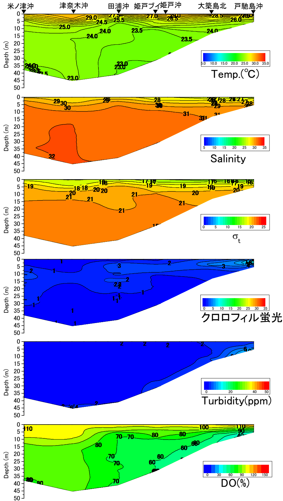
戸馳島沖から米ノ津沖の水温(°C)、塩分、密度( \sigma_t )、クロロフィル蛍光強度、濁度、溶存酸素飽和度(DO%)の鉛直面図(鹿児島県水産技術開発センターの調査による)(2016年8月3日)
