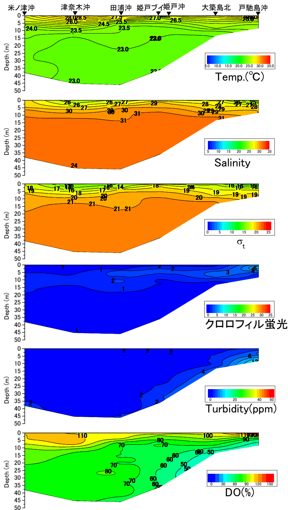
戸馳島沖から米ノ津沖の水温(°C)、塩分、密度( \sigma_t )、クロロフィル蛍光強度、濁度、溶存酸素飽和度(DO%)の鉛直面図(熊本県水産研究センターの調査による)(2016年7月25日)
