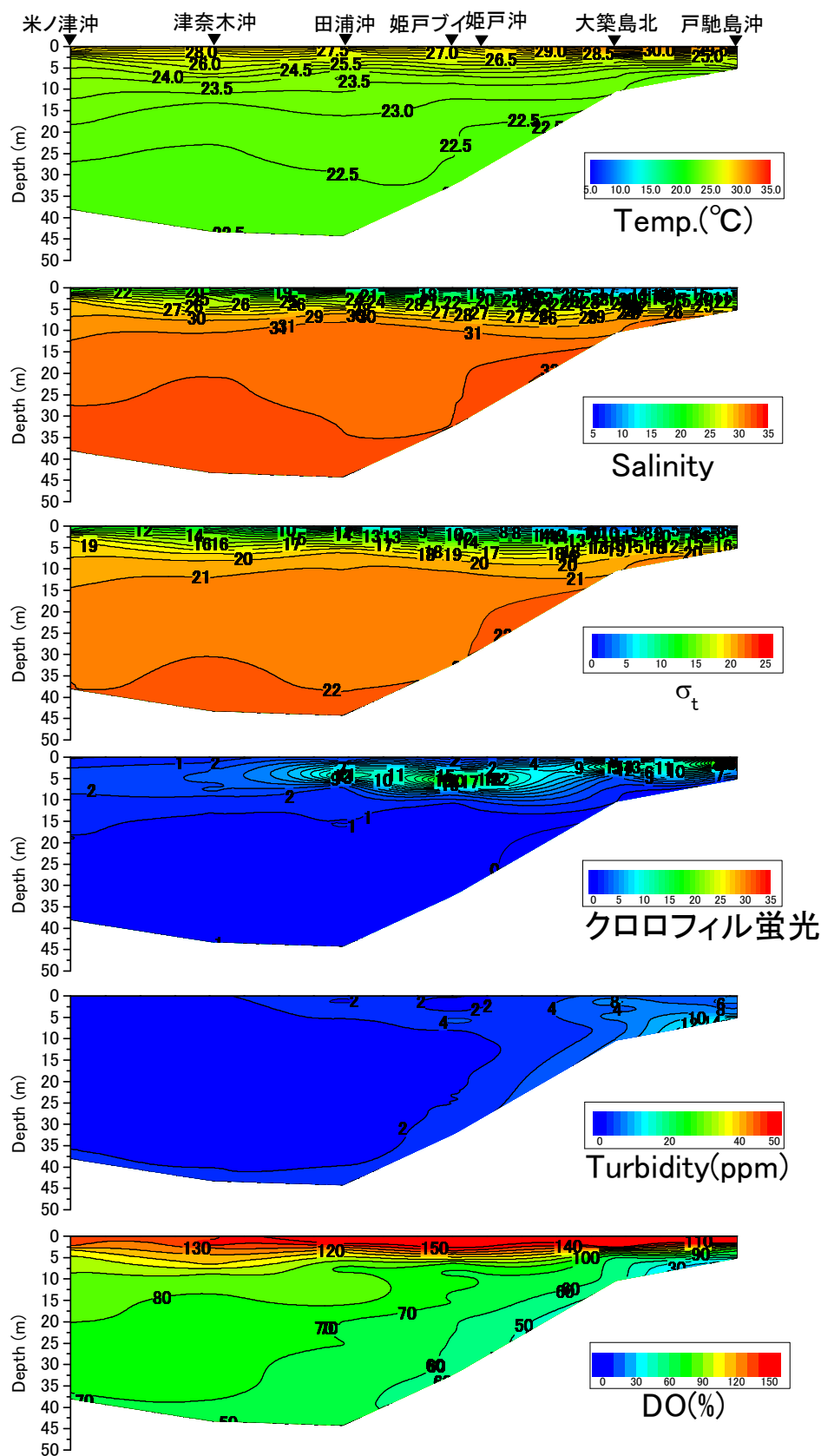
戸馳島沖から米ノ津沖の水温(°C)、塩分、密度( \sigma_t )、クロロフィル蛍光強度、濁度、溶存酸素飽和度(DO%)の鉛直面図(熊本県水産研究センターの調査による)(2016年7月19日)
