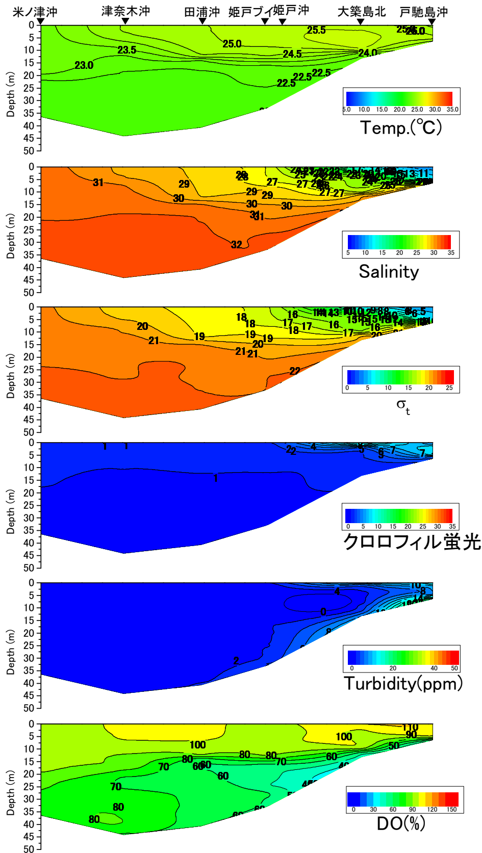
戸馳島沖から米ノ津沖の水温(°C)、塩分、密度( \sigma_t )、クロロフィル蛍光強度、濁度、溶存酸素飽和度(DO%)の鉛直面図(鹿児島県水産技術開発センターの調査による)(2016年7月13日)
