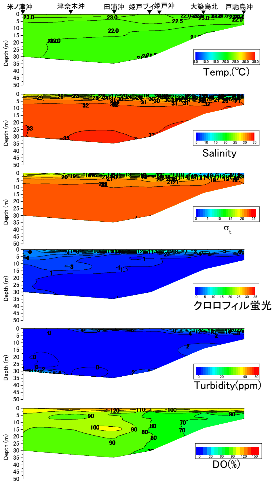
戸馳島沖から米ノ津沖の水温(°C)、塩分、密度( \sigma_t )、クロロフィル蛍光強度、濁度、溶存酸素飽和度(DO%)の鉛直面図(東町漁業協同組合の調査による) (2016年6月29日)
