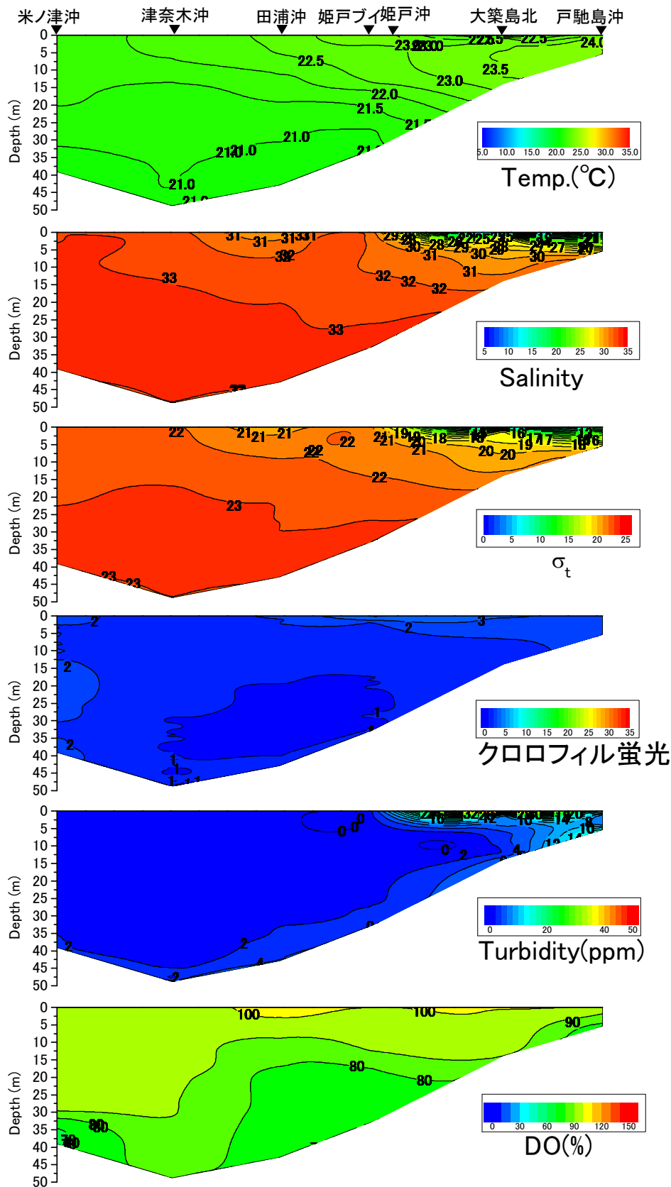
戸馳島沖から米ノ津沖の水温(°C)、塩分、密度( \sigma_t )、クロロフィル蛍光強度、濁度、溶存酸素飽和度(DO%)の鉛直面図(鹿児島県水産技術開発センターの調査による)(2016年6月21日)
