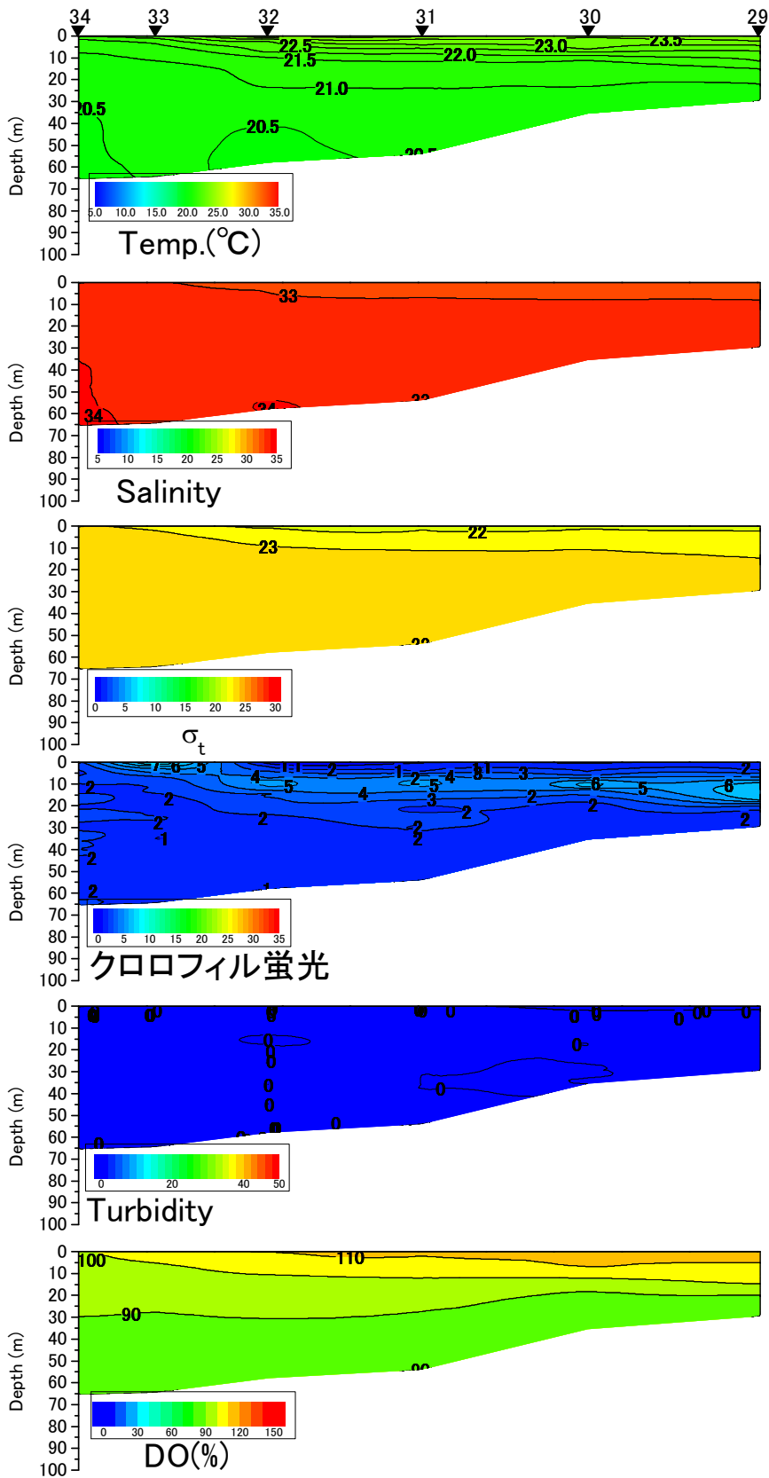
八代海西ラインの水温(°C)、塩分、密度( \sigma_t )、クロロフィル蛍光強度、濁度、溶存酸素飽和度(DO%)の鉛直面図(国土交通省の調査による) (2016年6月15日)
