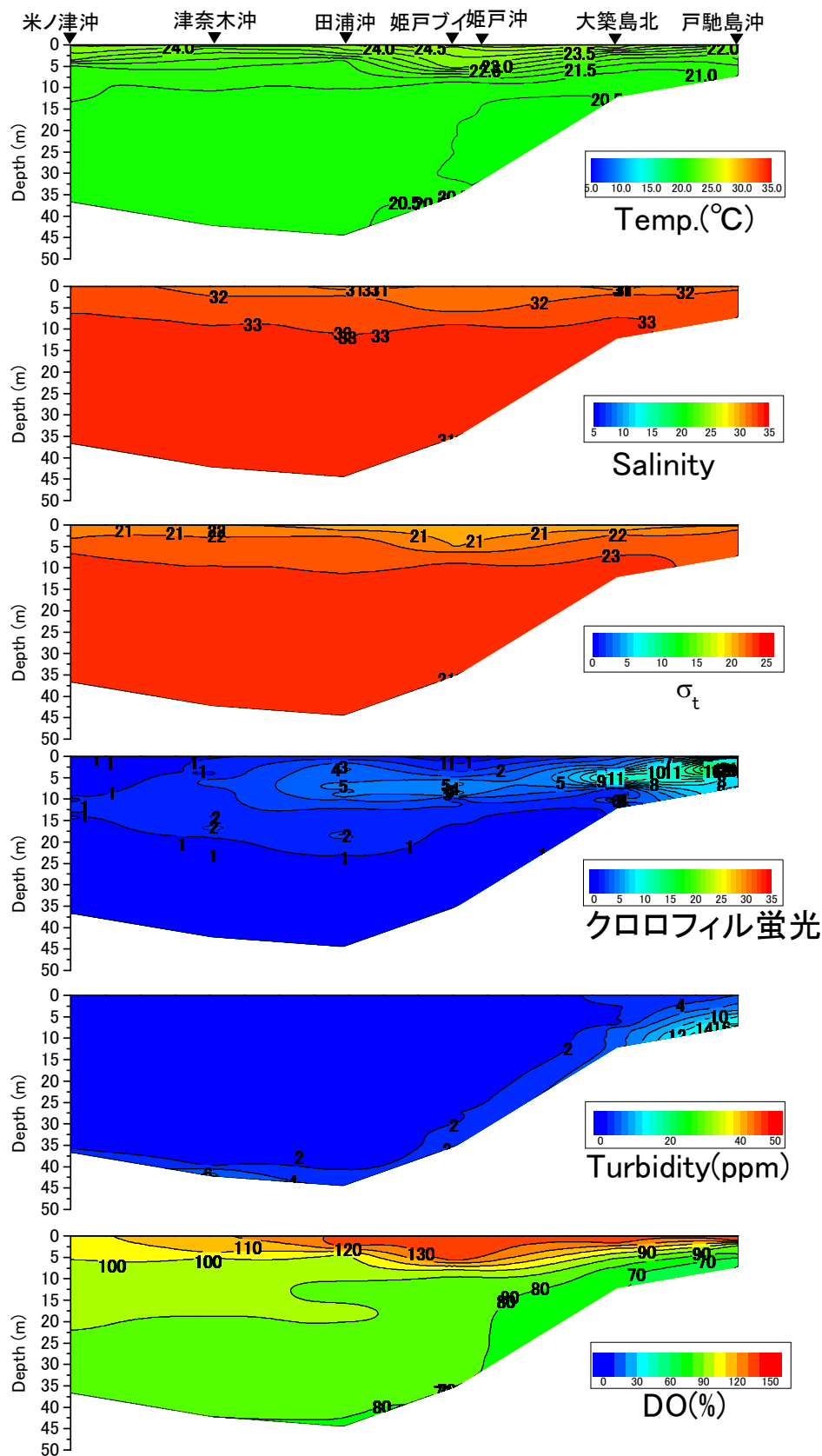
戸馳島沖から米ノ津沖の水温(°C)、塩分、密度( \sigma_t )、クロロフィル蛍光強度、濁度、溶存酸素飽和度(DO%)の鉛直面図(熊本県水産研究センターの調査による)(2016年6月14日)
