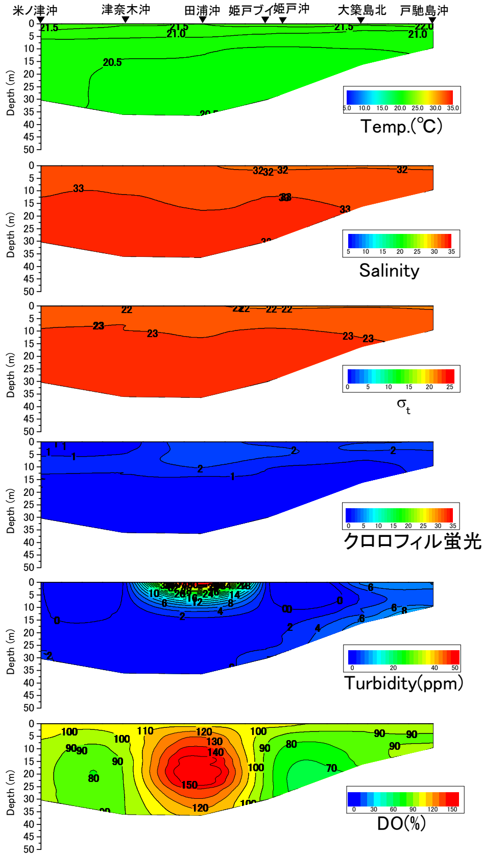
戸馳島沖から米ノ津沖の水温(°C)、塩分、密度( \sigma_t )、クロロフィル蛍光強度、濁度、溶存酸素飽和度(DO%)の鉛直面図(東町漁業協同組合の調査による) (2016年6月7日)
