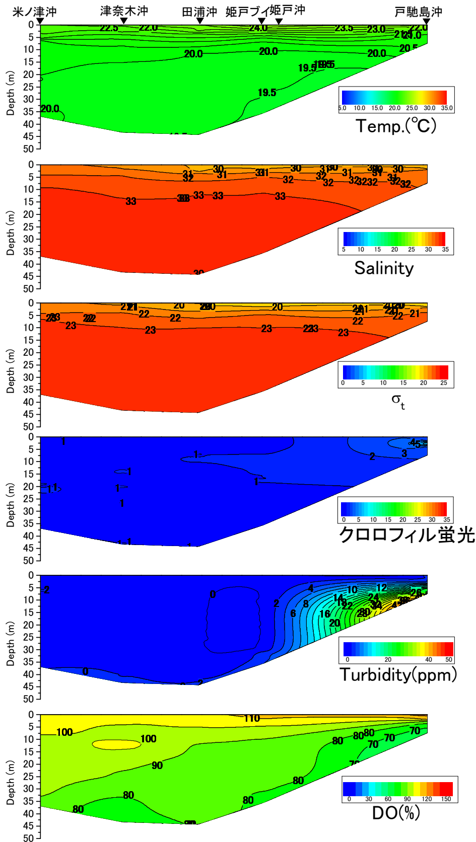
戸馳島沖から米ノ津沖の水温(°C)、塩分、密度( \sigma_t )、クロロフィル蛍光強度、濁度、溶存酸素飽和度(DO%)の鉛直面図(熊本県水産研究センターの調査による)(2016年5月31日)
