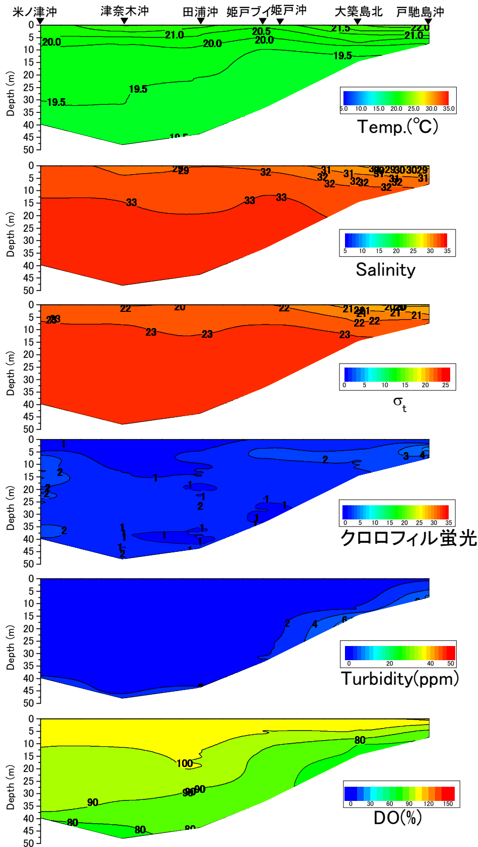
戸馳島沖から米ノ津沖の水温(°C)、塩分、密度( \sigma_t )、クロロフィル蛍光強度、濁度、溶存酸素飽和度(DO%)の鉛直面図(鹿児島県水産技術開発センターの調査による)(2016年5月24日)
