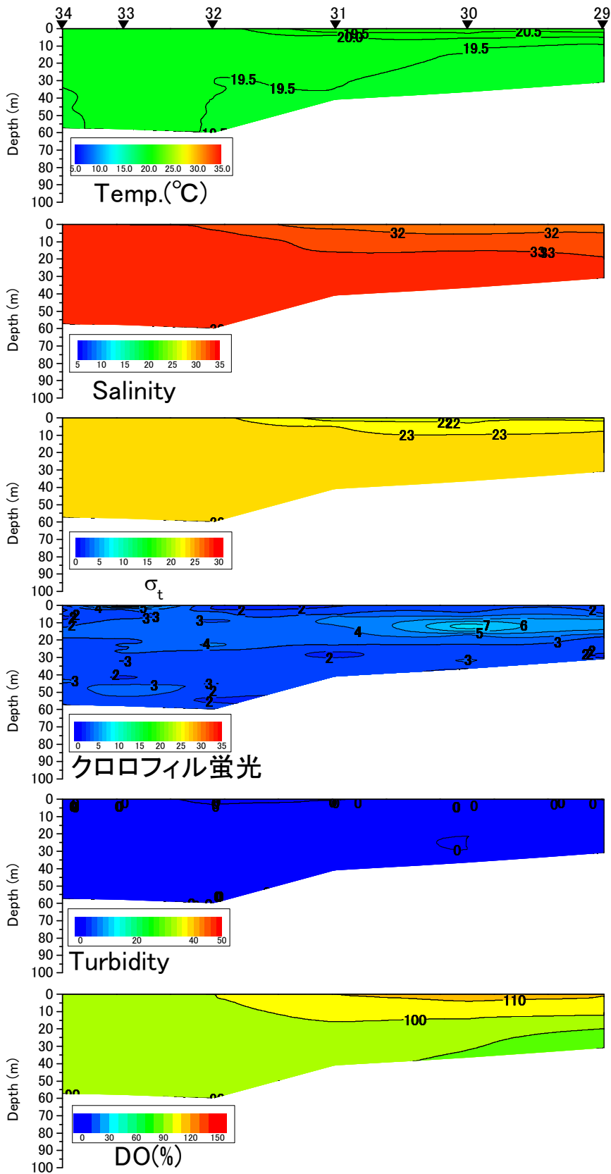
八代海西ラインの水温(°C)、塩分、密度( \sigma_t )、クロロフィル蛍光強度、濁度、溶存酸素飽和度(DO%)の鉛直面図(国土交通省の調査による) (2016年5月20日)
