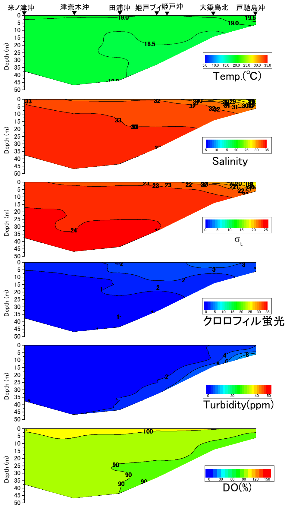
戸馳島沖から米ノ津沖の水温(°C)、塩分、密度( \sigma_t )、クロロフィル蛍光強度、濁度、溶存酸素飽和度(DO%)の鉛直面図(鹿児島県水産技術開発センターの調査による)(2016年5月10日)
