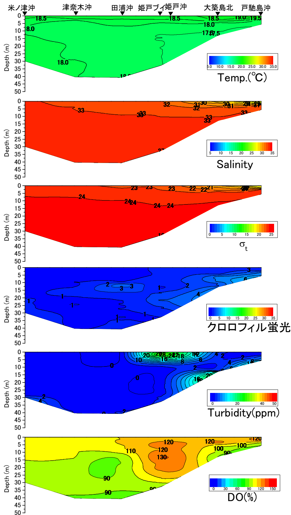
戸馳島沖から米ノ津沖の水温(°C)、塩分、密度( \sigma_t )、クロロフィル蛍光強度、濁度、溶存酸素飽和度(DO%)の鉛直面図(東町漁業協同組合の調査による) (2016年5月2日)
