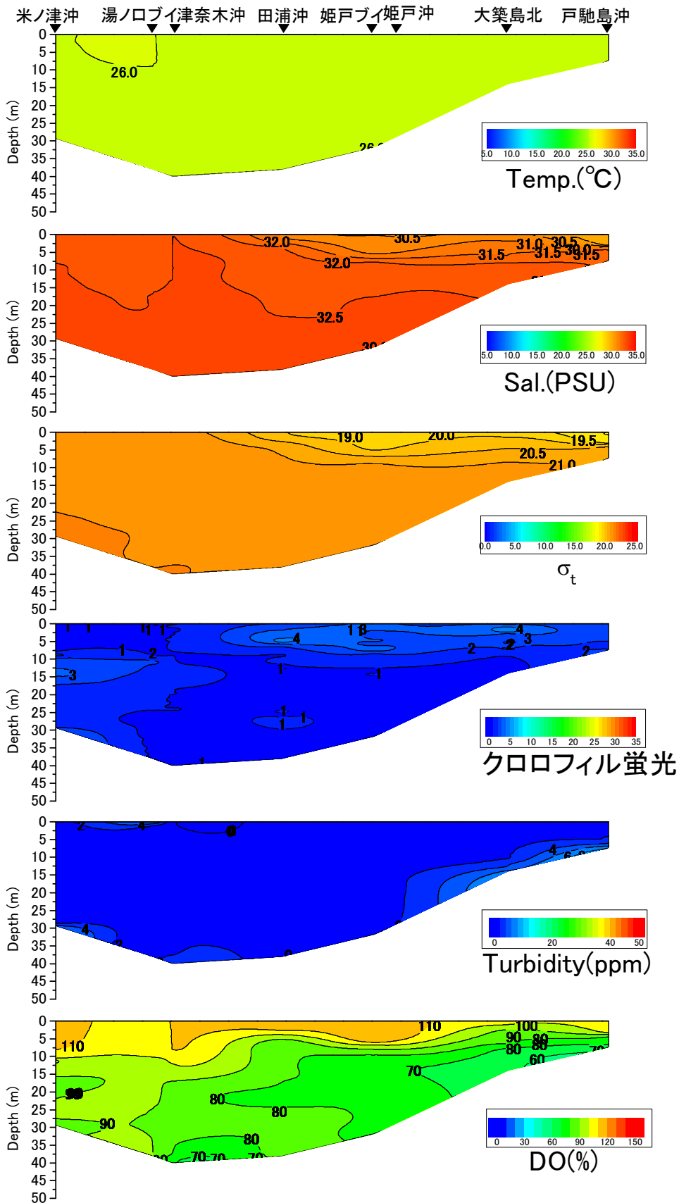
戸馳島沖から米ノ津沖の水温(°C)、塩分、密度( \sigma_t )、クロロフィル蛍光強度、濁度、溶存酸素飽和度(DO%)の鉛直面図(東町漁業協同組合の調査による) (2014年9月17日)
