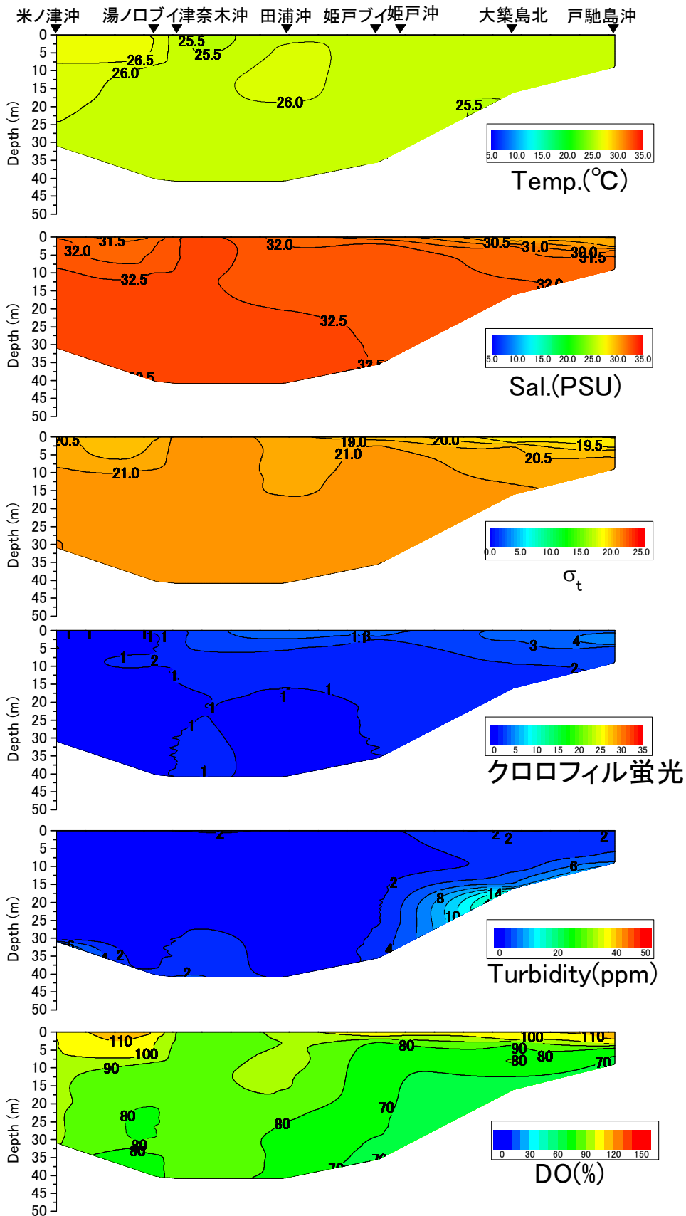
戸馳島沖から米ノ津沖の水温(°C)、塩分、密度( \sigma_t )、クロロフィル蛍光強度、濁度、溶存酸素飽和度(DO%)の鉛直面図(東町漁業協同組合の調査による) (2014年9月11日)
