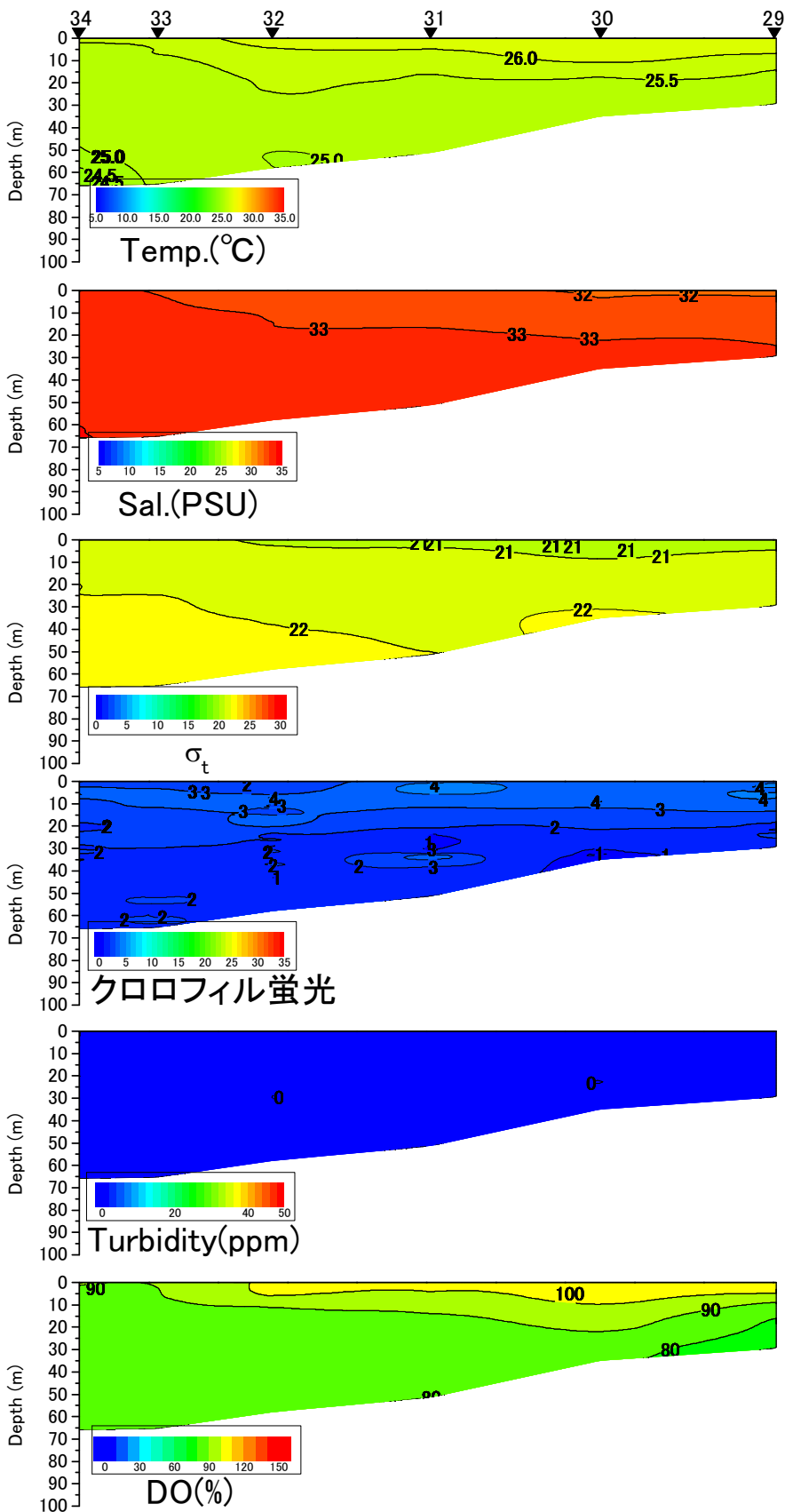
八代海西ラインの水温(°C)、塩分、密度( \sigma_t )、クロロフィル蛍光強度、濁度、溶存酸素飽和度(DO%)の鉛直面図(国土交通省の調査による) (2014年9月4日)
