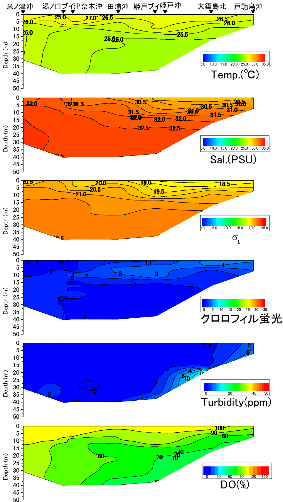
戸馳島沖から米ノ津沖の水温(°C)、塩分、密度( \sigma_t )、クロロフィル蛍光強度、濁度、溶存酸素飽和度(DO%)の鉛直面図(東町漁業協同組合の調査による) (2014年8月28日)
