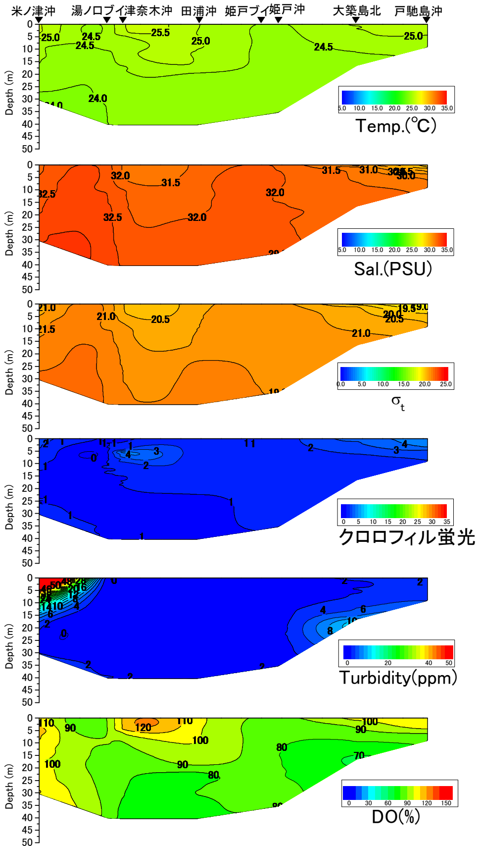
戸馳島沖から米ノ津沖の水温(°C)、塩分、密度( \sigma_t )、クロロフィル蛍光強度、濁度、溶存酸素飽和度(DO%)の鉛直面図(東町漁業協同組合の調査による) (2014年8月12日)
