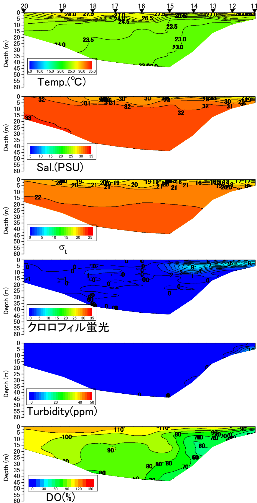
八代海中央ラインの水温(°C)、塩分、密度( \sigma_t )、クロロフィル蛍光強度、濁度、溶存酸素飽和度(DO%)の鉛直面図(国土交通省の調査による) (2014年7月30日)
