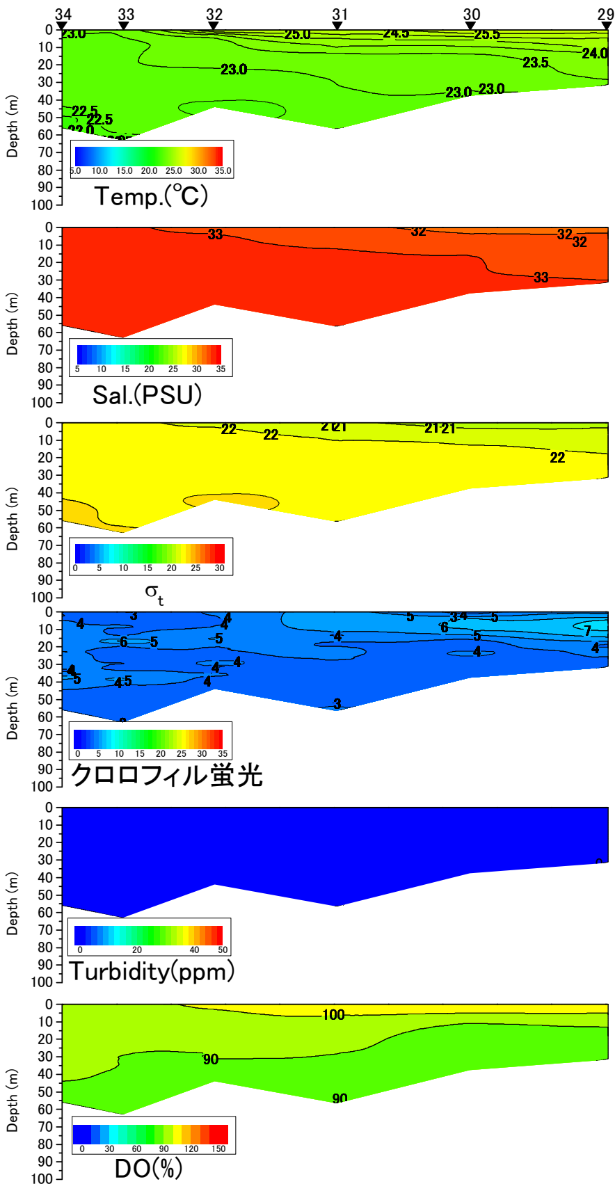
八代海西ラインの水温(°C)、塩分、密度( \sigma_t )、クロロフィル蛍光強度、濁度、溶存酸素飽和度(DO%)の鉛直面図(国土交通省の調査による) (2014年7月30日)
