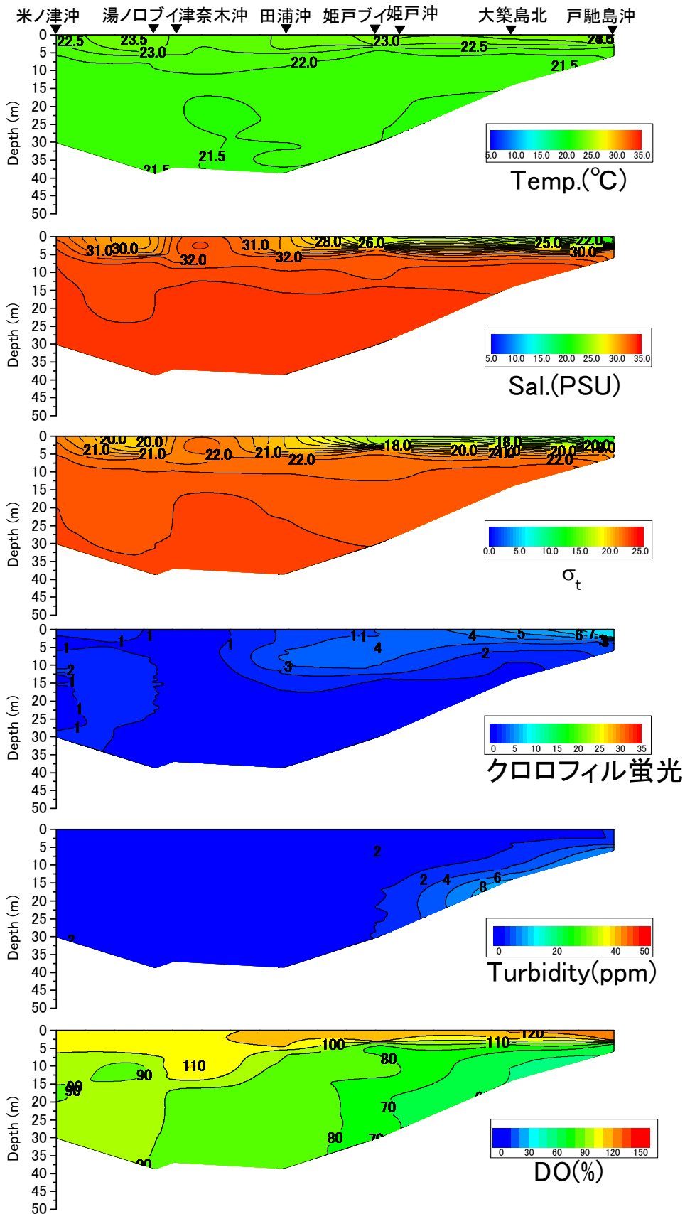
戸馳島沖から米ノ津沖の水温(°C)、塩分、密度( \sigma_t )、クロロフィル蛍光強度、濁度、溶存酸素飽和度(DO%)の鉛直面図(東町漁業協同組合の調査による) (2014年7月3日)
