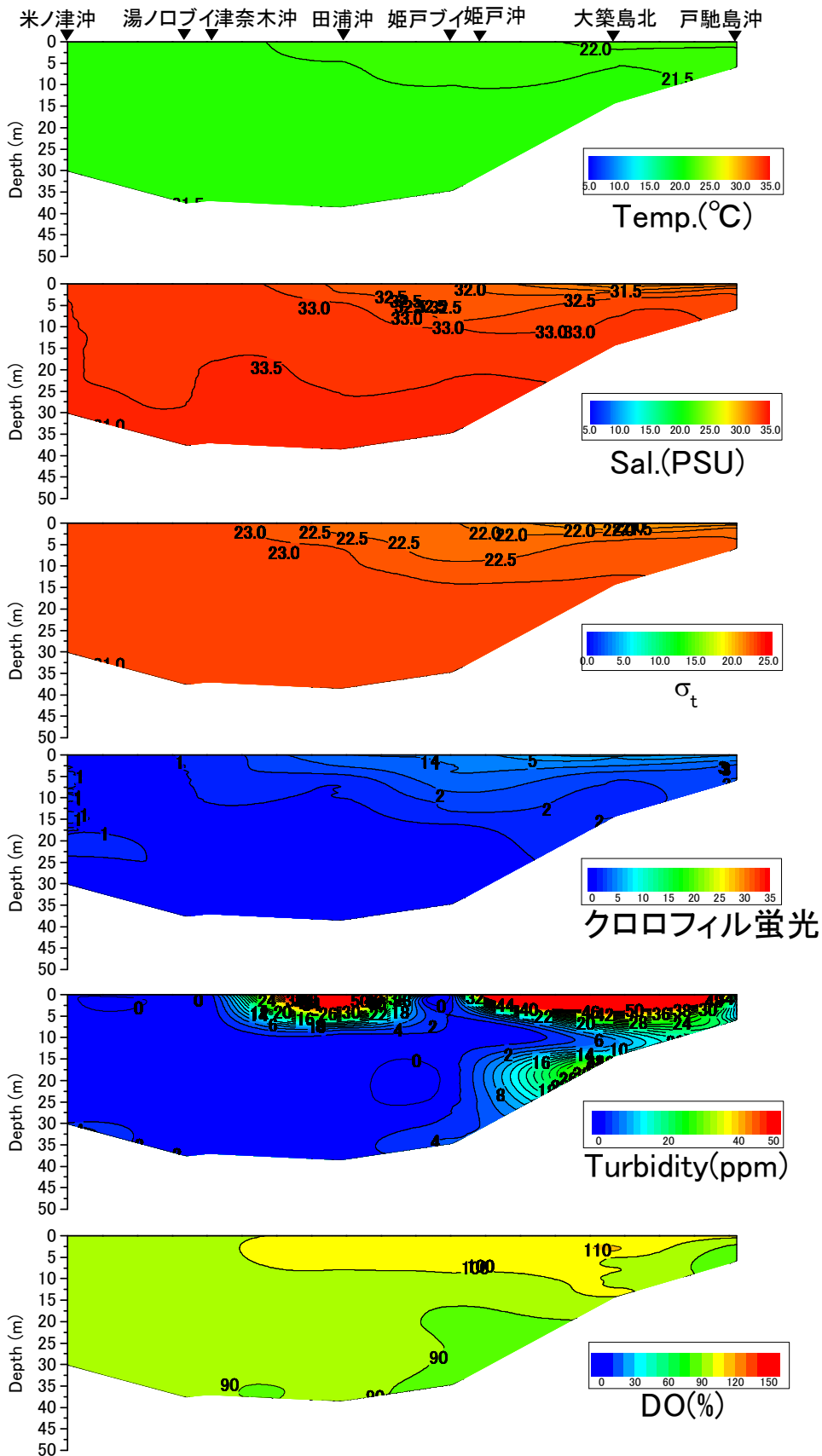
戸馳島沖から米ノ津沖の水温(°C)、塩分、密度( \sigma_t )、クロロフィル蛍光強度、濁度、溶存酸素飽和度(DO%)の鉛直面図(東町漁業協同組合の調査による) (2014年6月19日)
