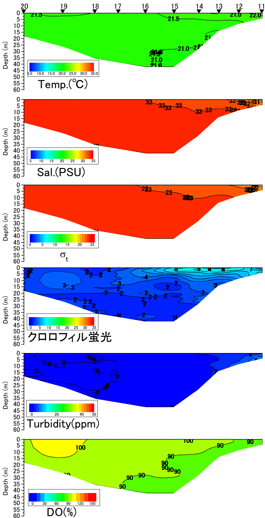
八代海中央ラインの水温(°C)、塩分、密度( \sigma_t )、クロロフィル蛍光強度、濁度、溶存酸素飽和度(DO%)の鉛直面図(国土交通省の調査による) (2014年6月19日)
