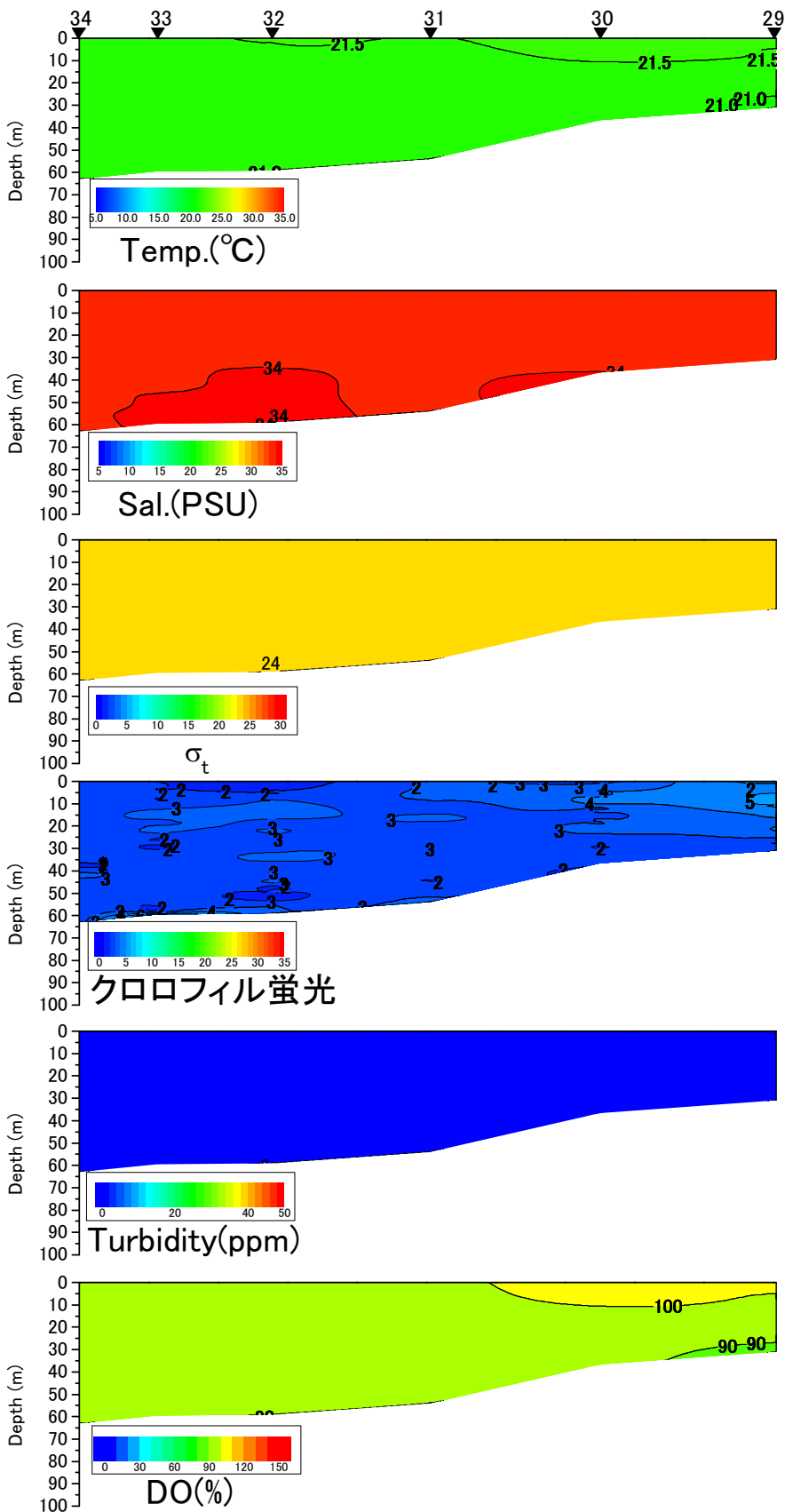
八代海西ラインの水温(°C)、塩分、密度( \sigma_t )、クロロフィル蛍光強度、濁度、溶存酸素飽和度(DO%)の鉛直面図(国土交通省の調査による) (2014年6月13日)
