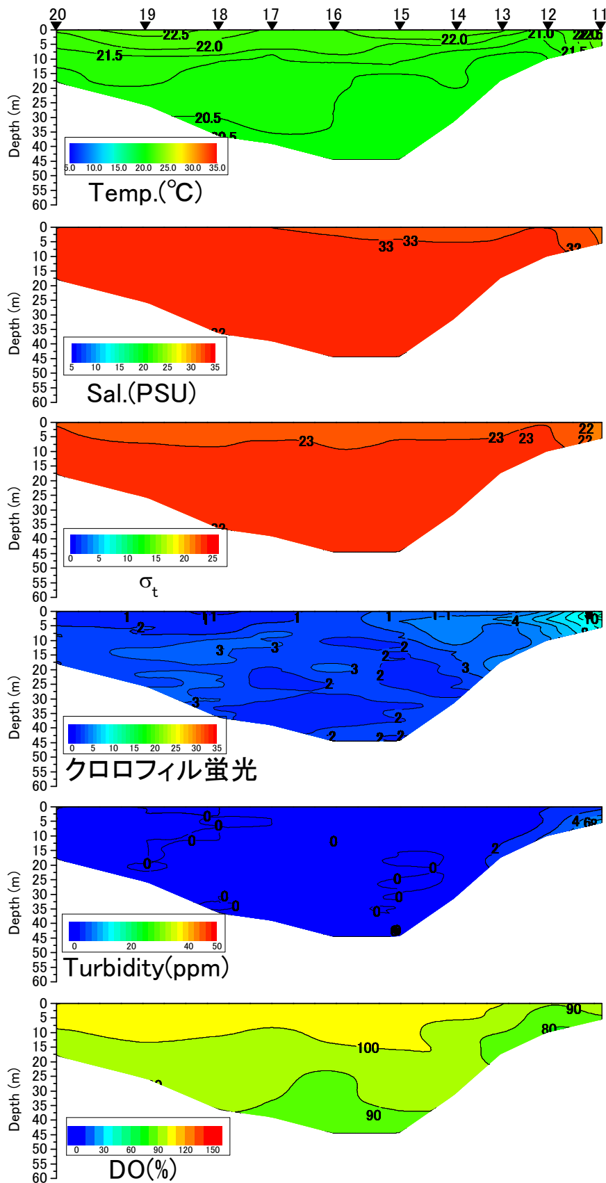
八代海中央ラインの水温(°C)、塩分、密度( \sigma_t )、クロロフィル蛍光強度、濁度、溶存酸素飽和度(DO%)の鉛直面図(国土交通省の調査による) (2014年6月13日)
