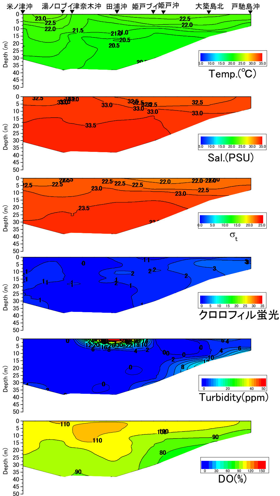
戸馳島沖から米ノ津沖の水温(°C)、塩分、密度( \sigma_t )、クロロフィル蛍光強度、濁度、溶存酸素飽和度(DO%)の鉛直面図(東町漁業協同組合の調査による) (2014年6月12日)
