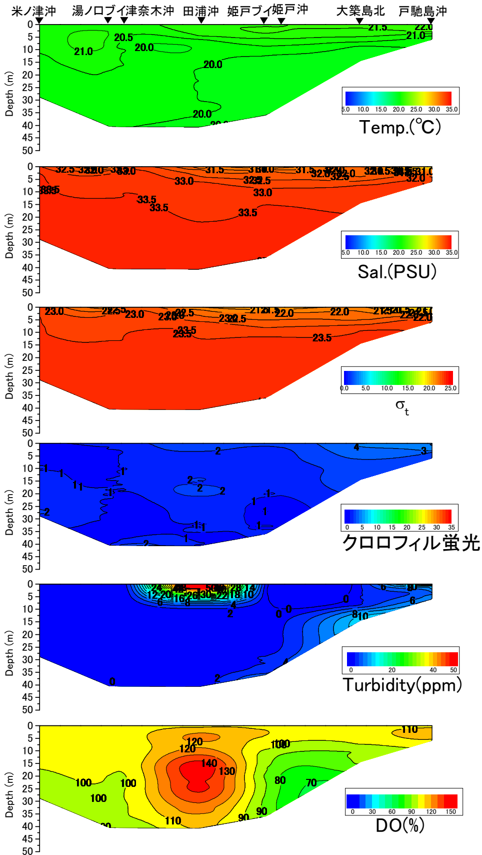
戸馳島沖から米ノ津沖の水温(°C)、塩分、密度( \sigma_t )、クロロフィル蛍光強度、濁度、溶存酸素飽和度(DO%)の鉛直面図(東町漁業協同組合の調査による) (2014年6月5日)
