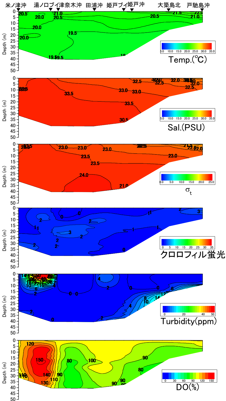
戸馳島沖から米ノ津沖の水温(°C)、塩分、密度( \sigma_t )、クロロフィル蛍光強度、濁度、溶存酸素飽和度(DO%)の鉛直面図(東町漁業協同組合の調査による) (2014年5月30日)
