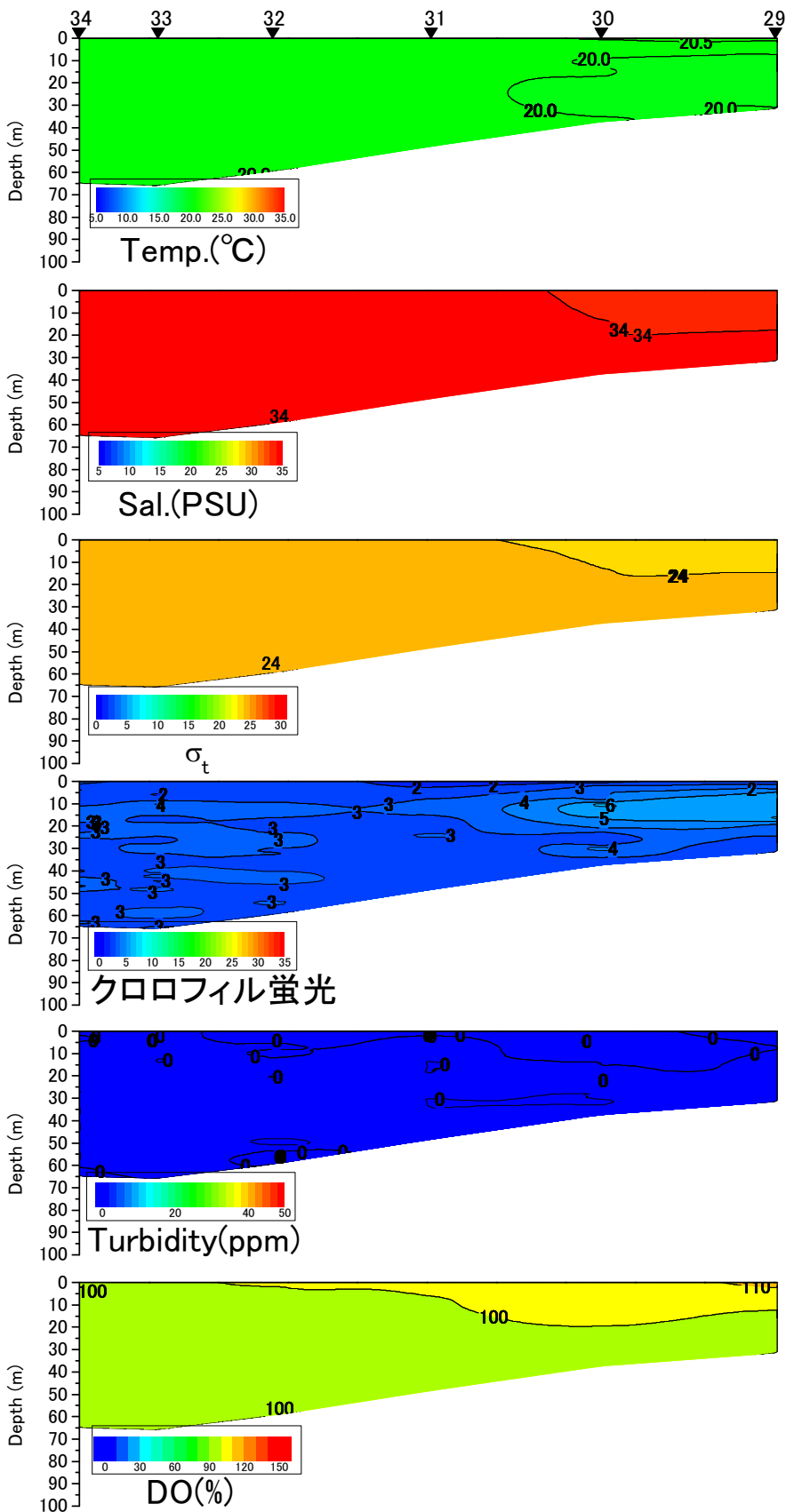
八代海西ラインの水温(°C)、塩分、密度( \sigma_t )、クロロフィル蛍光強度、濁度、溶存酸素飽和度(DO%)の鉛直面図(国土交通省の調査による) (2014年5月30日)
