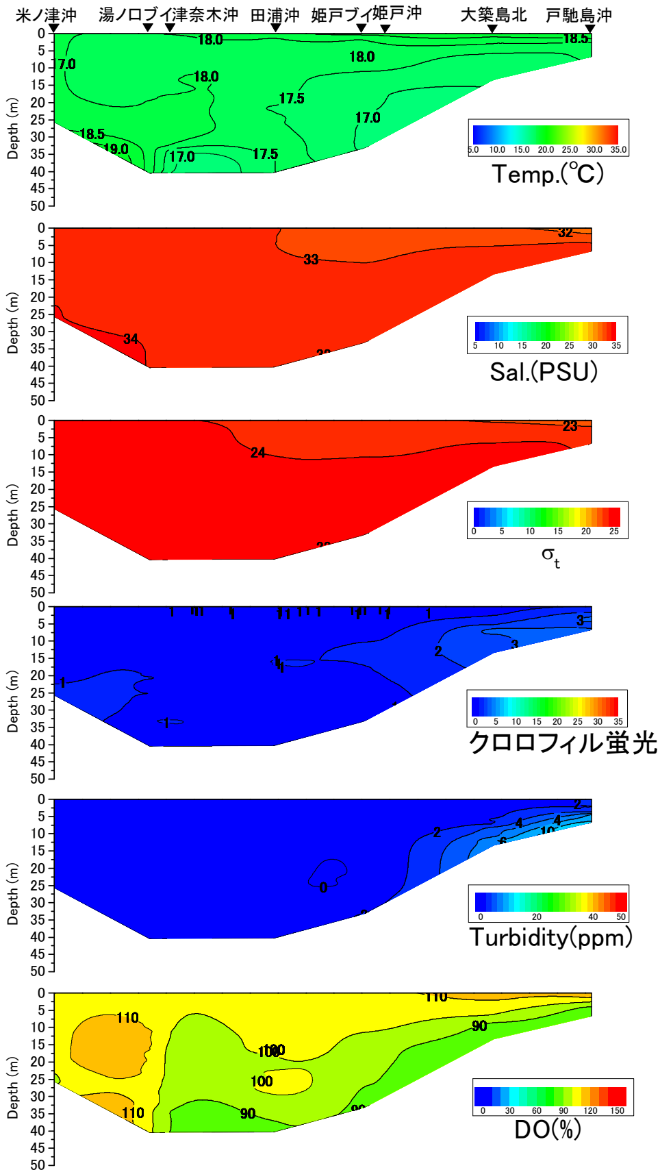
戸馳島沖から米ノ津沖の水温(°C)、塩分、密度( \sigma_t )、クロロフィル蛍光強度、濁度、溶存酸素飽和度(DO%)の鉛直面図(東町漁業協同組合の調査による) (2014年5月8日)
