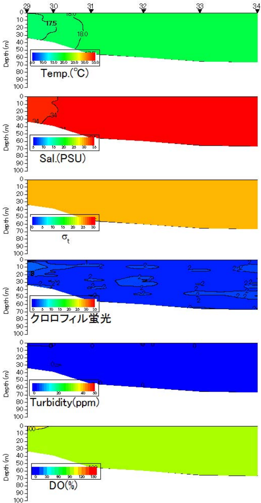
八代海西ラインの水温(°C)、塩分、密度( \sigma_t )、クロロフィル蛍光強度、濁度、溶存酸素飽和度(DO%)の鉛直面図(国土交通省の調査による) (2014年5月1日)
