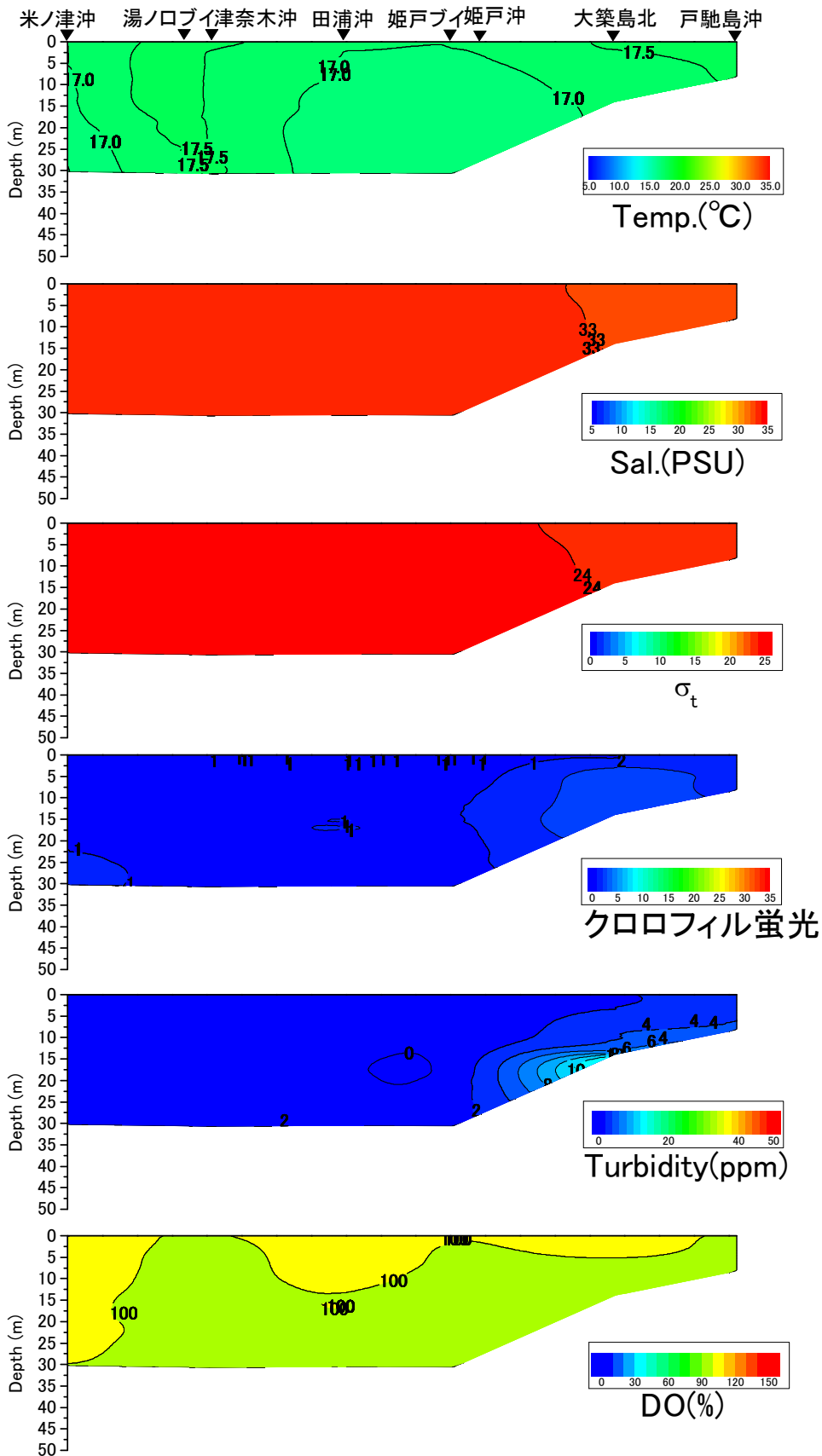
戸馳島沖から米ノ津沖の水温(°C)、塩分、密度( \sigma_t )、クロロフィル蛍光強度、濁度、溶存酸素飽和度(DO%)の鉛直面図(東町漁業協同組合の調査による) (2014年5月1日)
