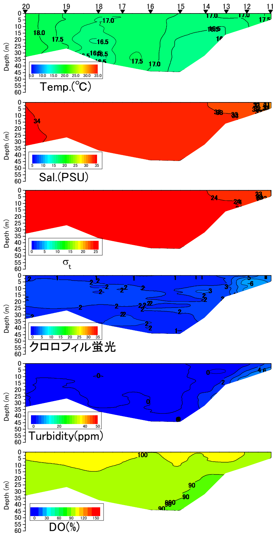
八代海中央ラインの水温(°C)、塩分、密度( \sigma_t )、クロロフィル蛍光強度、濁度、溶存酸素飽和度(DO%)の鉛直面図(国土交通省の調査による) (2014年5月1日)
