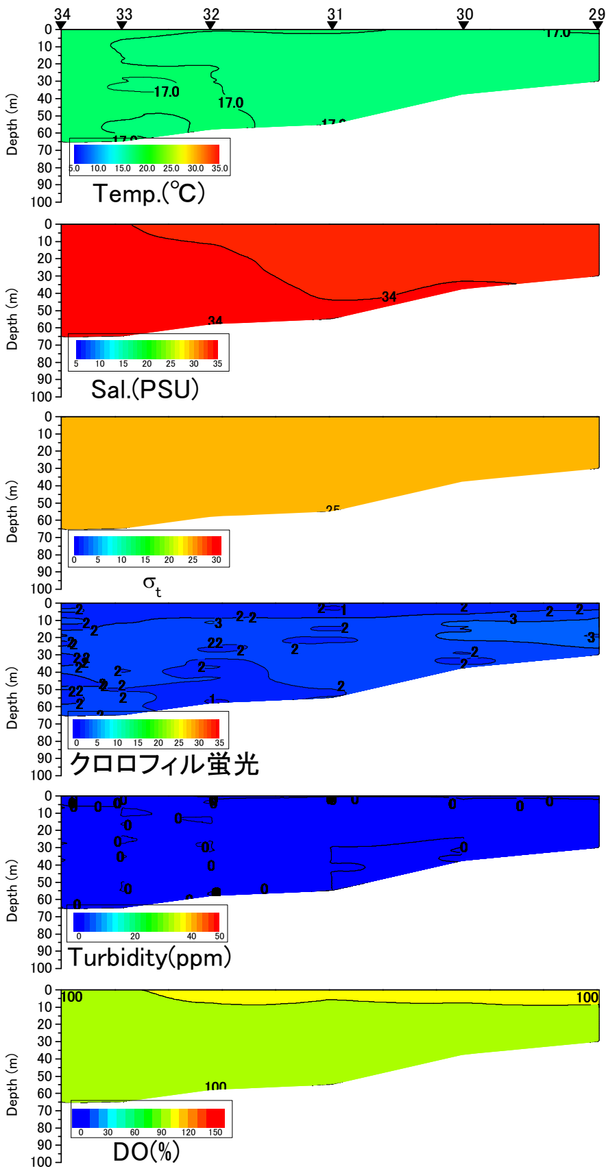
八代海西ラインの水温(°C)、塩分、密度( \sigma_t )、クロロフィル蛍光強度、濁度、溶存酸素飽和度(DO%)の鉛直面図(国土交通省の調査による) (2014年4月25日)
